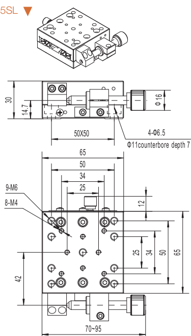
PSM25-65SL ▼
