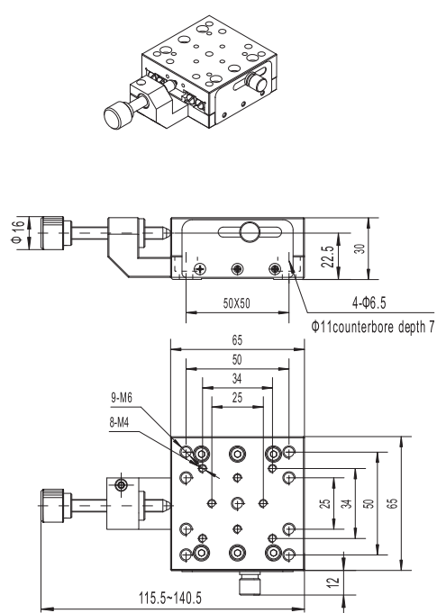
PSM25-65C ▼
